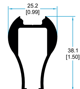
4611 TIRADOR REFUERZO
