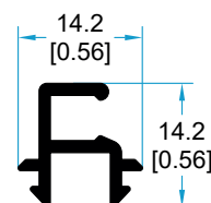
4610 ADAPTADOR MOSQUITERO
