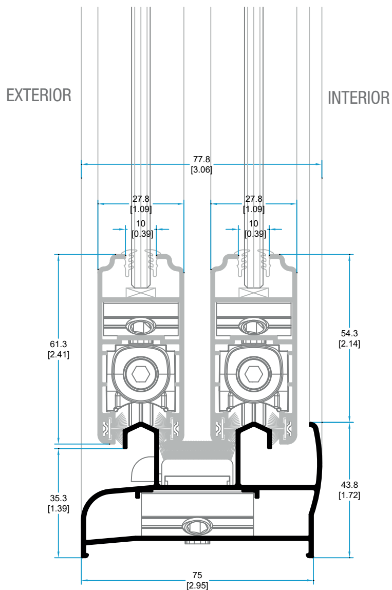
4601 MARCO PERIMETRAL
