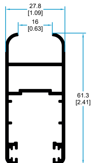
4615 HOJA PERIMETRAL PLAYA
