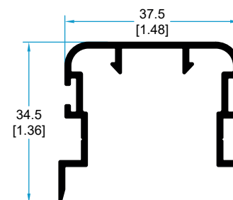
*64614 TAPA DOBLE HOJA CENTRAL
