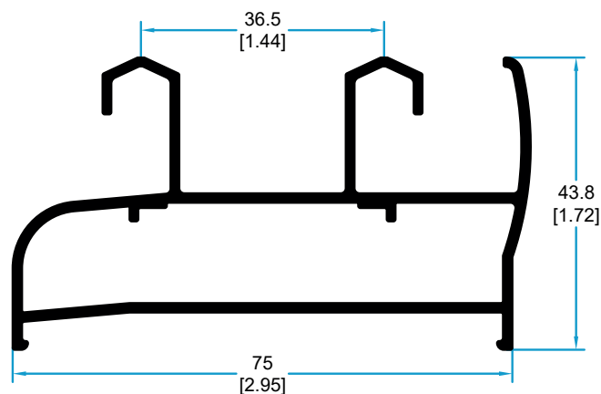
4601 MARCO PERIMETRAL
