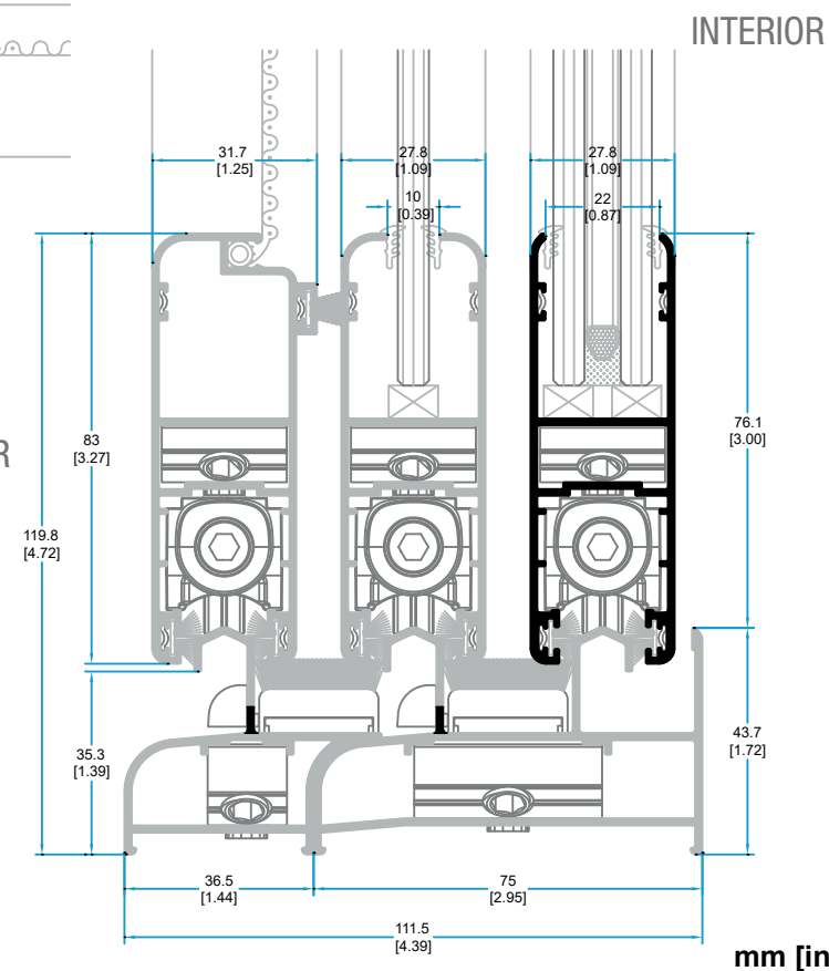
64621 HOJA PERIMETRAL DOBLE VIDRIO MONUMENTAL
