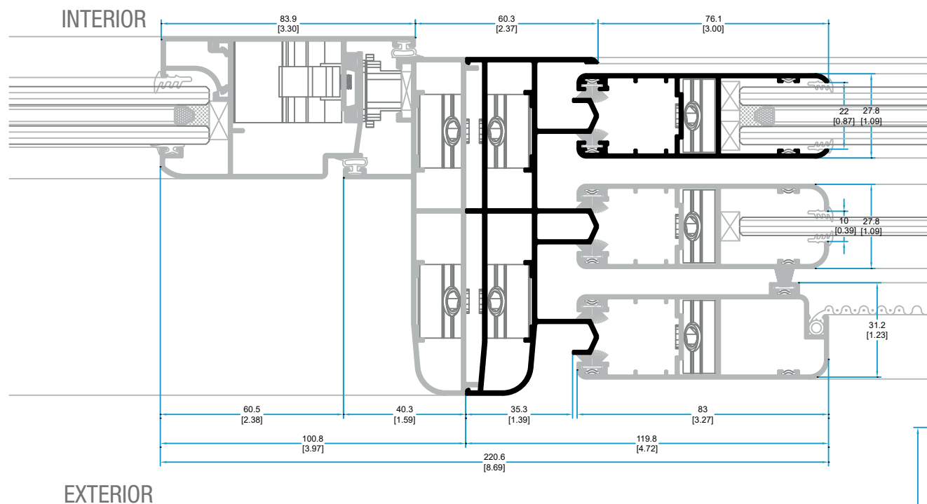
74632 MARCO PERIMETRAL TRES RIELES RECTO
